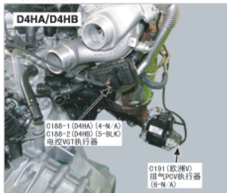
33. 发动机后左
