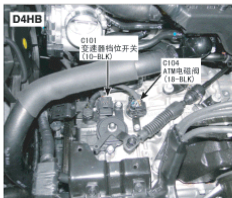
34. 变速器顶部
