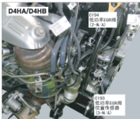
32. 发动机后右
